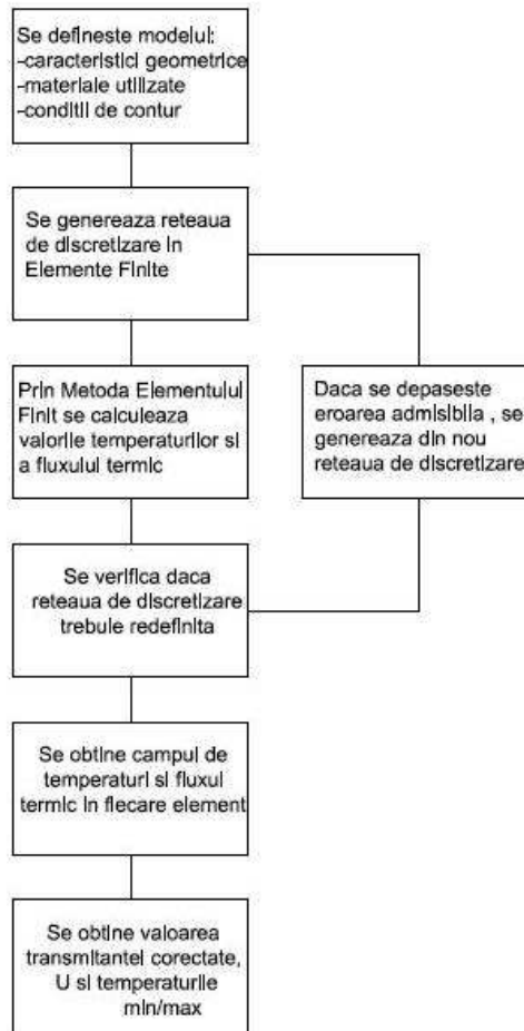
Fig. 2.5 Pașii de lucru necesari în analiza numerică a unui detaliu constructiv în programul THERM
