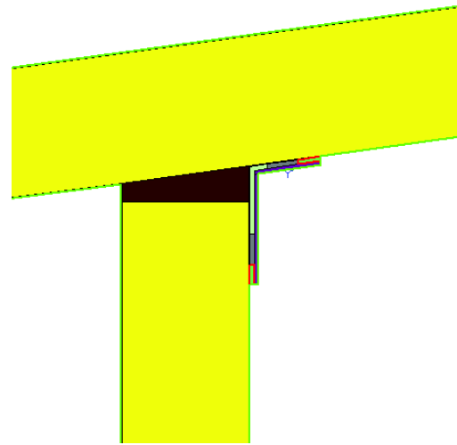
Fig. 3.18 Detaliu modelare geometrică
