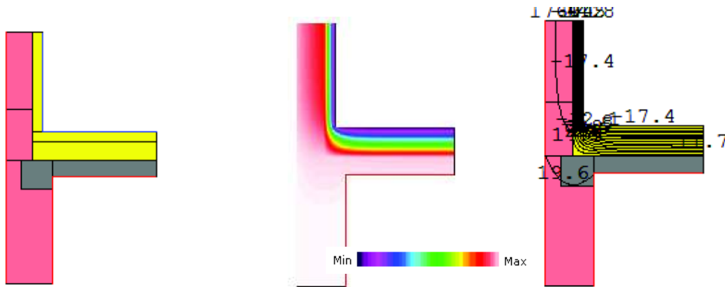
Fig. 6.55 Detaliu int. per. neîncălzit casa scării cu planșeu din lemn, spre pod neîncălzit (a) Modelul geometric (b) Suprafețe izoterme (c) Linii izoterme
