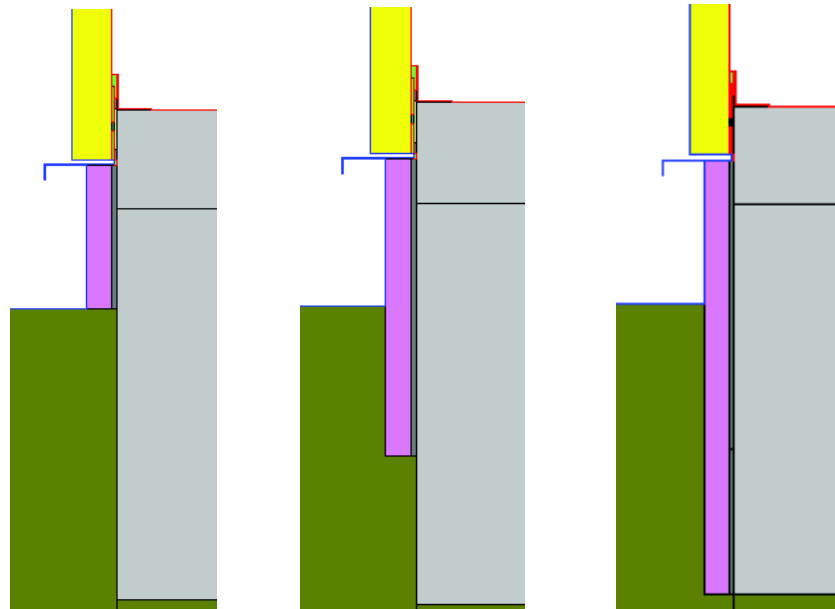
Fig. 3.45 Detalii de modelare geometrică pentru soluțiile de tip 2 – termoizolare soclu și fundație a) Soluția 2.a b) Soluția 2.b c) Soluția 2.c
