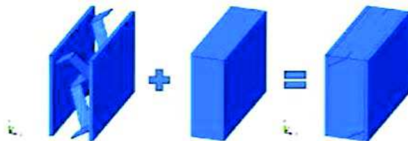
Fig. 2.8 Panou sandwich multifuncțional cu structură celulară expandată mecanic ExpaAsym, al cărui spațiu intracelular este umplut cu materiale stohastice [63]
