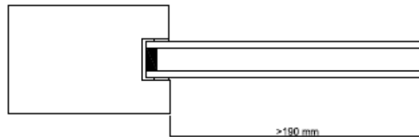
Fig. 3.4 Lungimea de secționare cu planuri adiabatic zona ferestre – specificații SR EN10077
