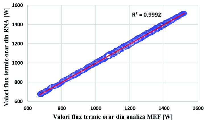
Fig. 5.3 Verificare performanță RNA: Regresie pentru rețeaua neuronală 2-10-30-1
