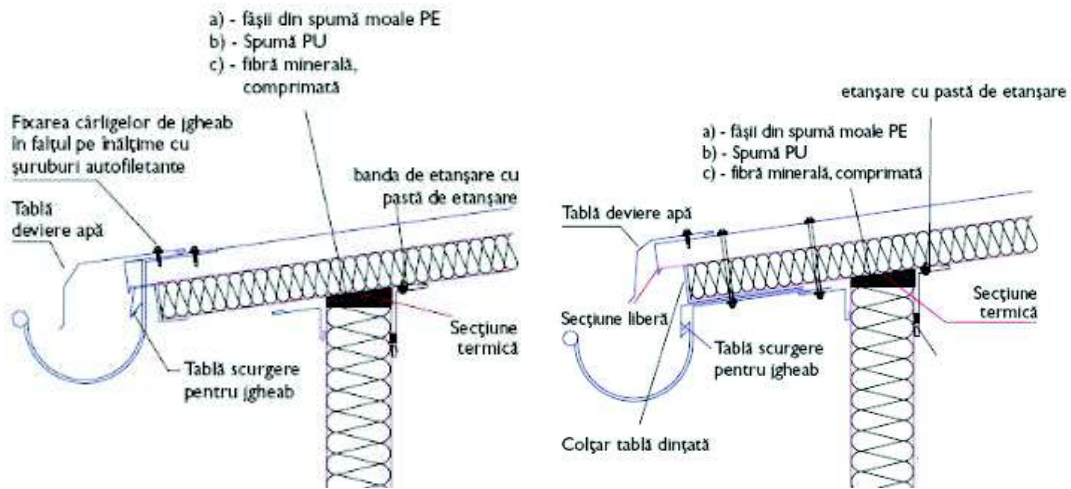
Fig. 2.16 Detalii de îmbinare panouri la streașină
