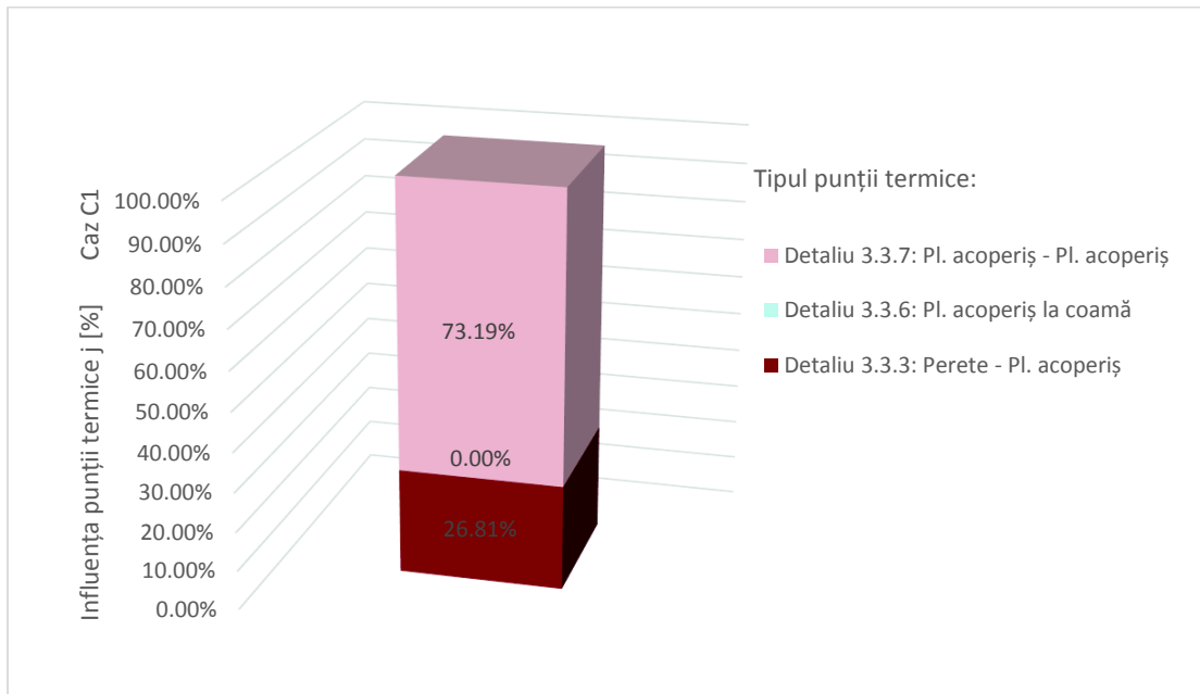
Fig. 3.56 Analiza influenței punților termice asupra planșeului acoperiș analizat – Caz C1
