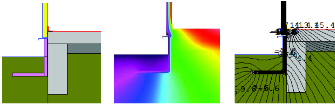
Fig. 3.46 Detalii de simulare numerică pentru soluția 2.c a) Detaliu modelare geometrică b) Suprafețe izoterme
