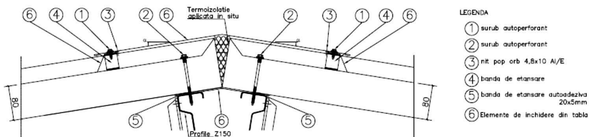
Fig. 3.33 Detaliu de îmbinare panouri acoperiș, la coamă
