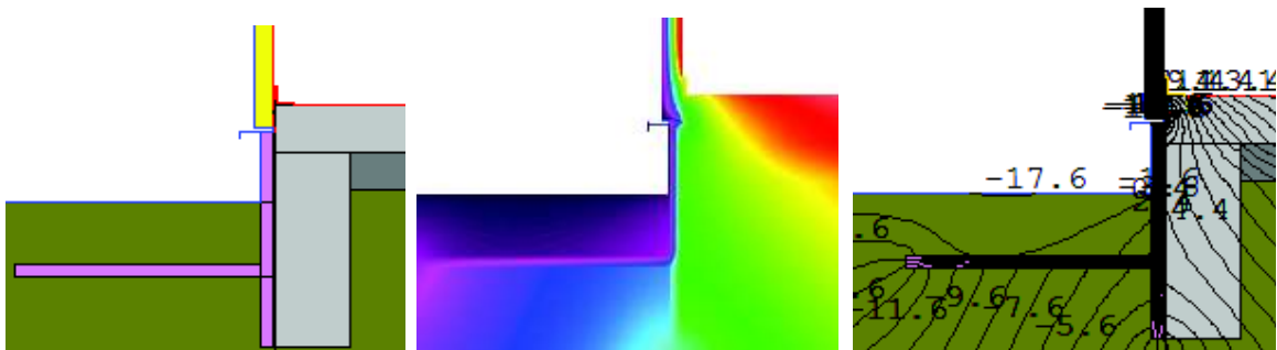
Fig. 3.49 Detalii de simulare numerică pentru soluția 2.g a) Detaliu modelare geometrică b) Suprafețe izoterme
