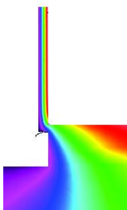
Fig. 3.32 Suprafețe izoterme detaliu 3.3.5.2
