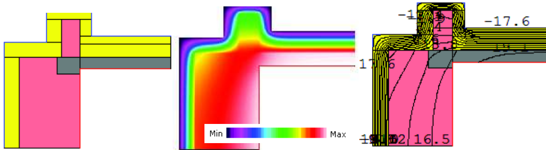
Fig. 6.54 Detaliu intersecție per. ext. P1 cu planșeu din lemn, sub pod, P11 (a) Modelul geometric (b) Suprafețe izoterme (c) Linii izoterme
