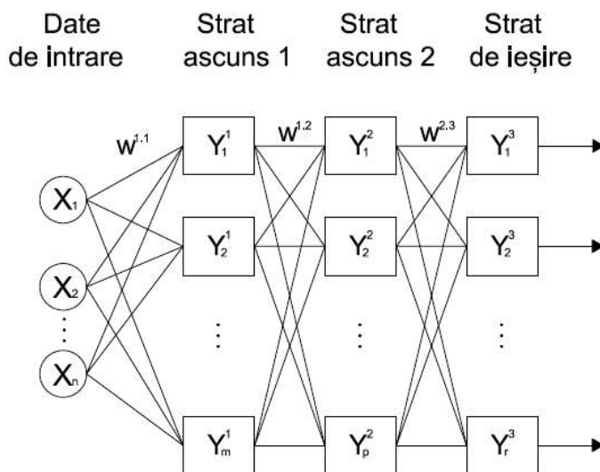
Fig. 5.1 Schema principală a unei rețele neuronale feedforward multistrat
