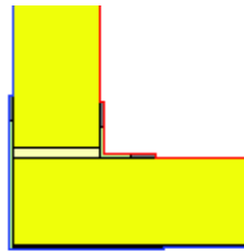
Fig. 3.6 Detaliu modelare geometrică îmbinare între panouri de perete - la colț
