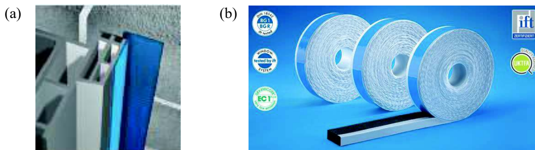
Fig. 6.18 Soluții propuse de etanșare a îmbinărilor tâmplărie fereastră/ ușă cu peretele exterior [160] (a) Benzi ISO Connect-Vario XD. Producător: ISO CHEMIE GmbH (b) Benzi precomprimare ISO BLOCO ONE
