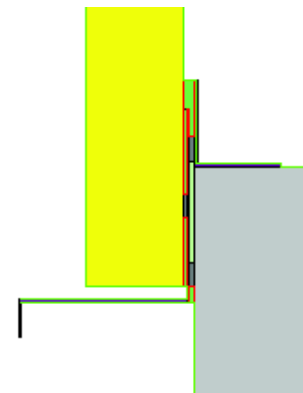
Fig. 3.26 Modelare geom. zone interstițiale
