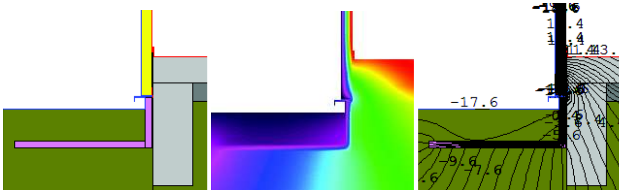
Fig. 3.47 Detalii de simulare numerică pentru soluția 2.d a) Detaliu modelare geometrică b) Suprafețe izoterme
