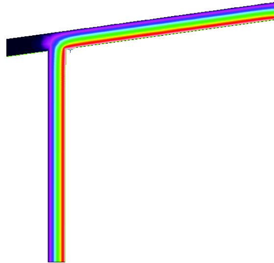
Fig. 3.20 Suprafețe izoterme detaliu 3.3.3
