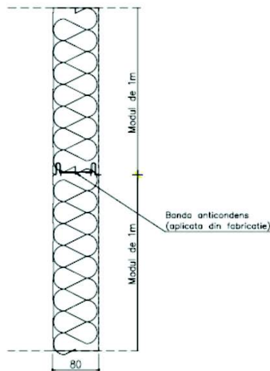
Fig. 3.9 Detaliu îmbinare orizontală panouri de perete
