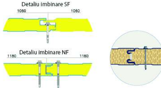
Fig. 2.15 Detalii îmbinare panouri de perete
