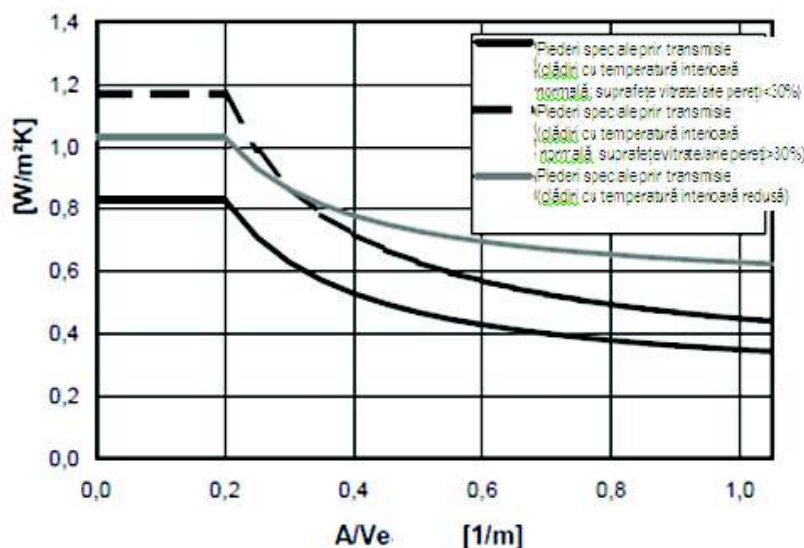
Fig. 2.4 Valori de referință ale coeficientului special de pierderi termice prin transmisie pentru clădirea de referință din sectorul terțiar în Germania
