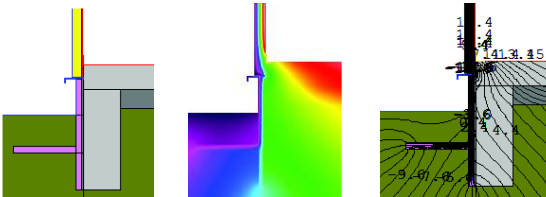
Fig. 3.48 Detalii de simulare numerică pentru soluția 2.f a) Detaliu modelare geometrică b) Suprafețe izoterme
