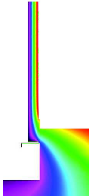
Fig. 3.28 Suprafețe izoterme detaliul 3.3.5.1
