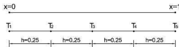
Fig. 4.3 Discretizarea modelului numeric în elemente finite
