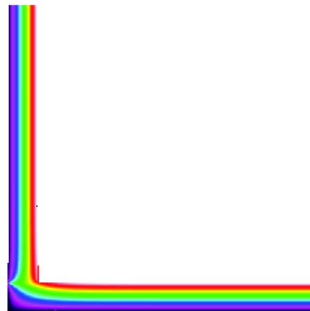
Fig. 3.8 Suprafețe izoterme detaliu 3.3.1
