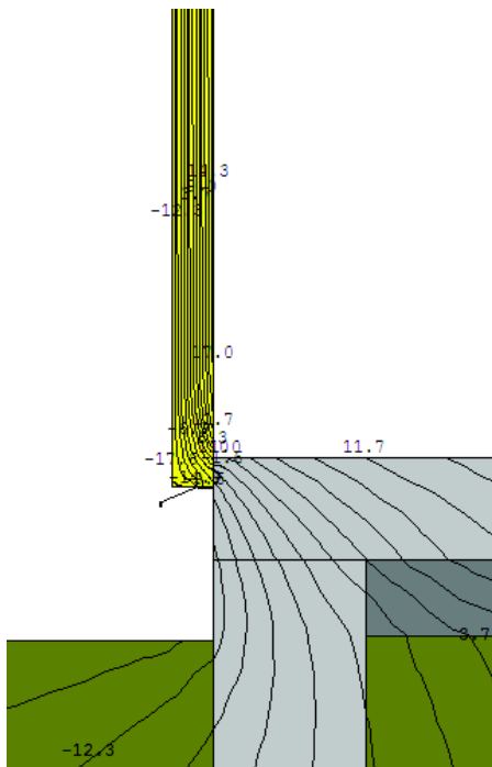
Fig. 3.31 Linii izoterme detaliu 3.3.5.2
