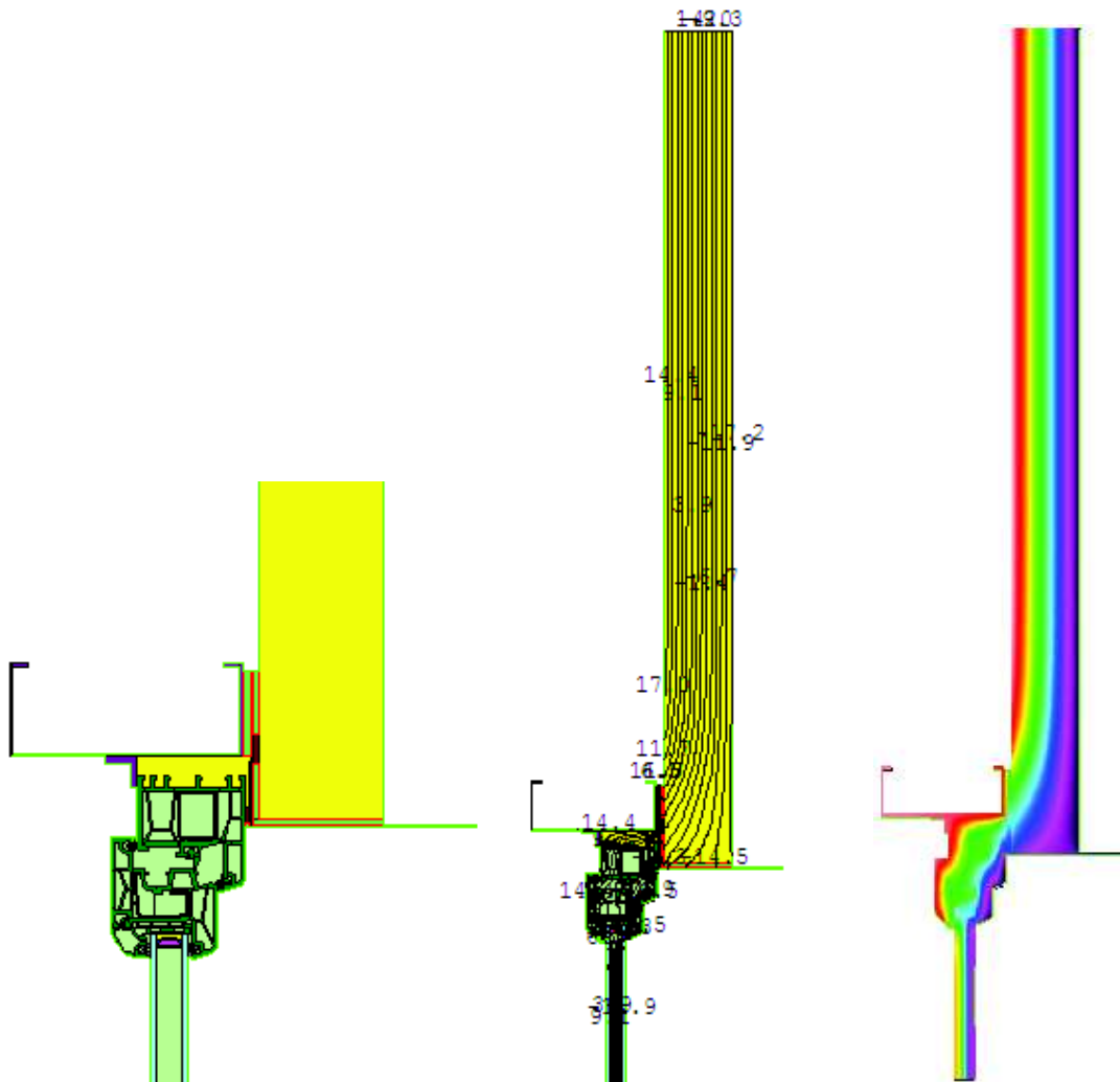
Fig. 3.22 Detaliu modelare geom. Fig. 3.23 Linii izoterme det. 3.3.4 Fig. 3.24 Suprafețe izoterme det. 3.3
